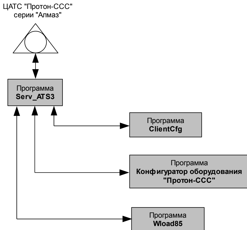
Рисунок 1.1 – Структурная схема ЦТО для ЦАТС "Протон-ССС" серии "Алмаз"
